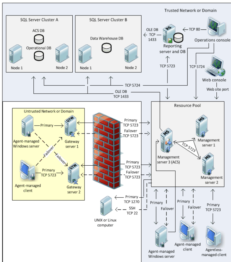
Figuur 20 SCOM topologie 8
