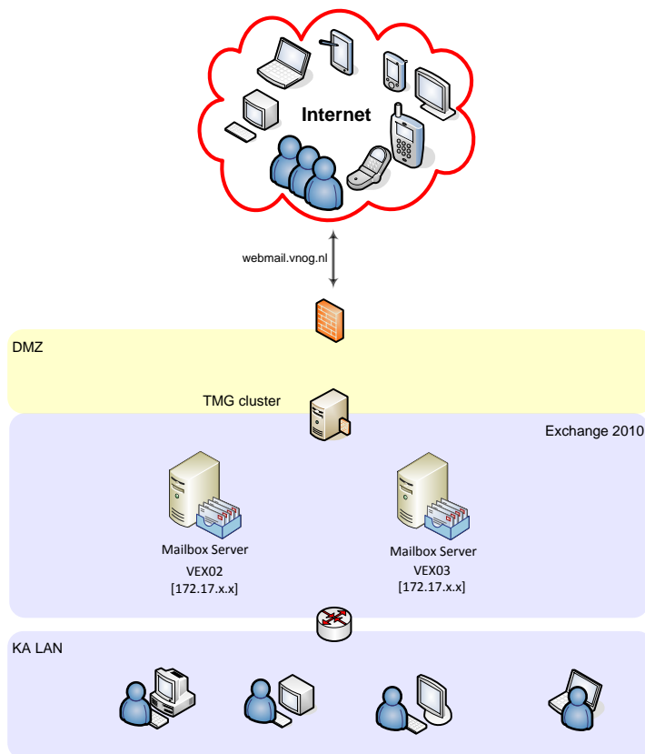
Figuur 12 Exchange infrastructuur
