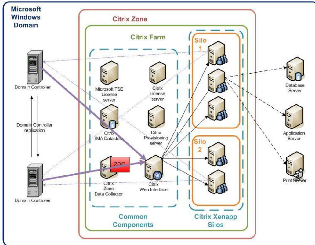
Figuur 16 Relatie Citrix en AD
