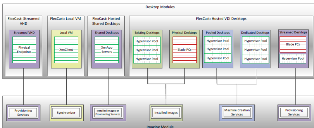
Figuur 14 FlexCast opties (Bron: Citrix)
